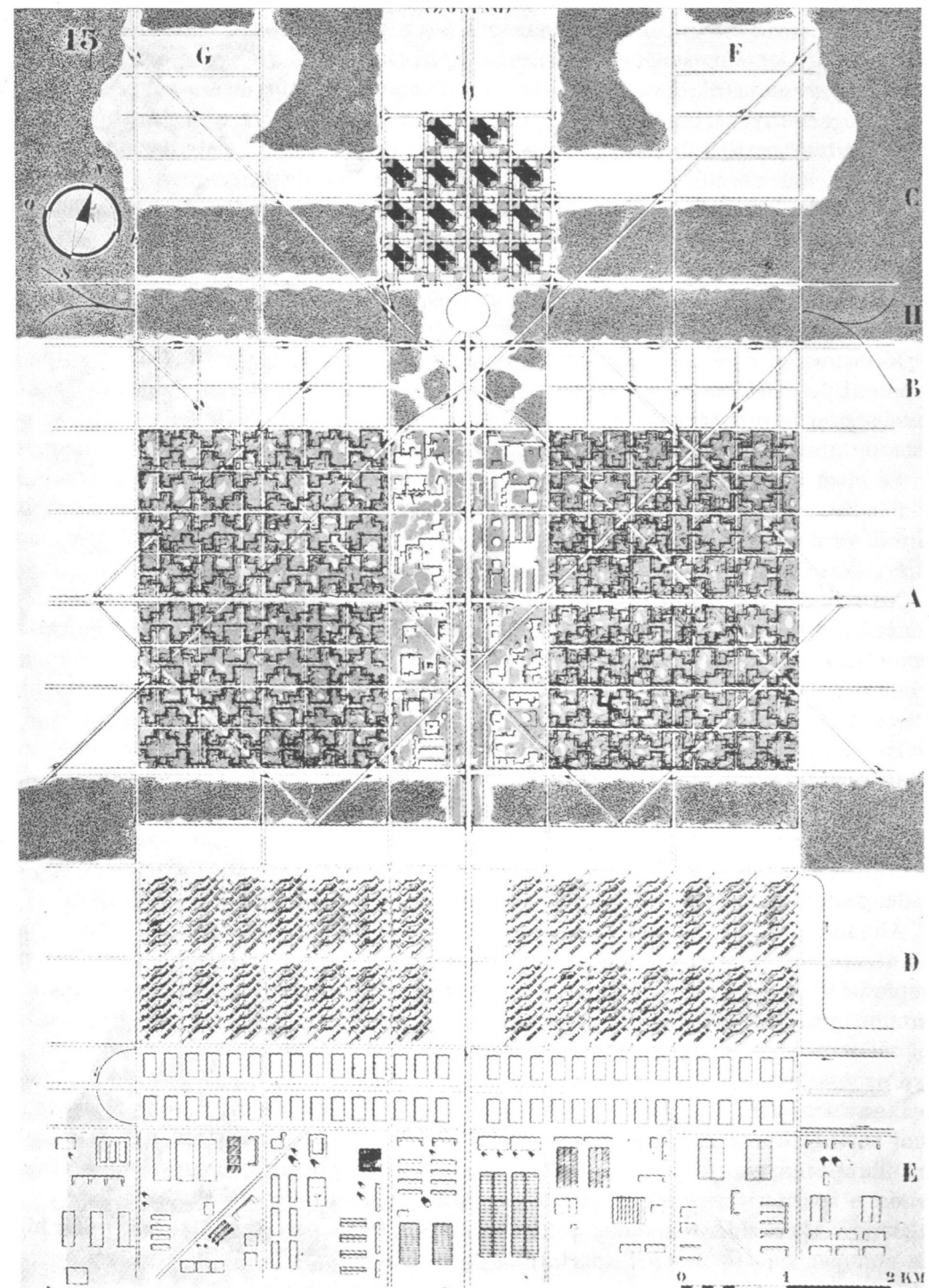
La planimetria della Ville Radieuse (Le Corbusier).
